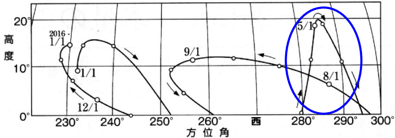
天文年鑑2015より→ 図3 日没時の水星の高度と方位角（東京での値）
