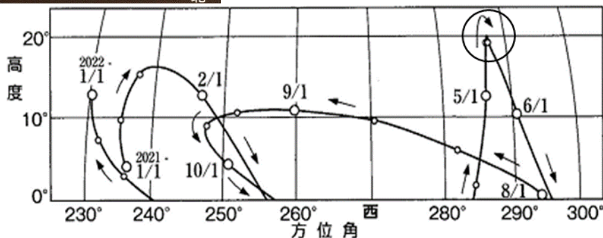
日没時の水星の高度と方位角(東京での値)
